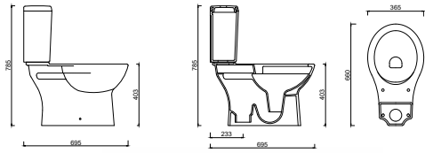
TR23KLZ00 TRIA RIMLESS DUVARA DAYALI KLOZET TR02RZV00 REZERVUAR TR00KRK48 KLOZET + REZERVUAR
