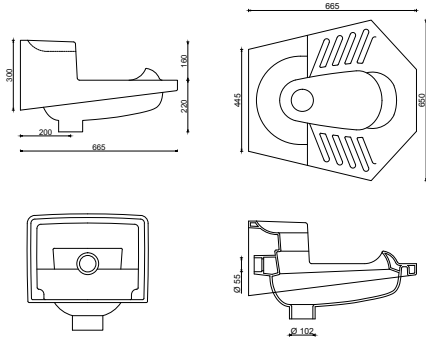
CV00HLT01 CAVALLETTA YENİ NESİL HELA TAŞI
