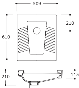
TP02HLT00 ÇEVRE YIKAMALI HELA TAŞI
