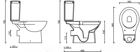
TR03KLZ00 TRIA RIMLESS DUVARA YARIM DAYALI KLOZET TR02RZV00 REZERVUAR
