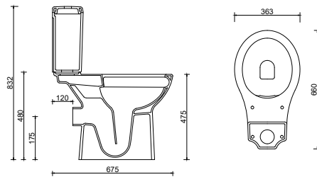
CA19KLZ00 CARMINA RIMLESS ENGELLİ KLOZET (ARKA ÇIKIŞLI) CA09RZV00 REZERVUAR
