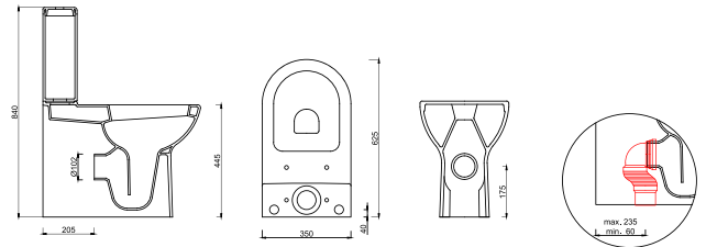
CA17KLZ00 CARMINA ENGELLİ KLOZETİ CA01RZV00 REZERVUAR
